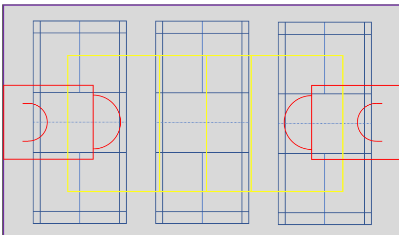
Figuur 2 Indeling vloer gymzaal 26.000 x 15.400 mm
