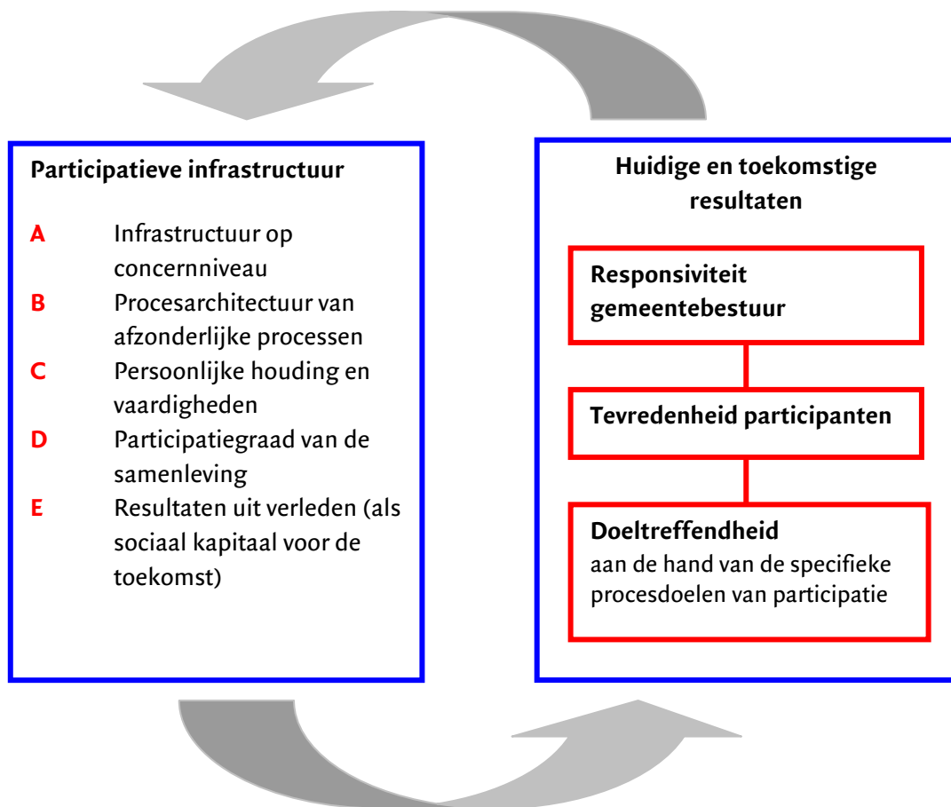
Afbeelding 2.1: het onderzoeksmodel
